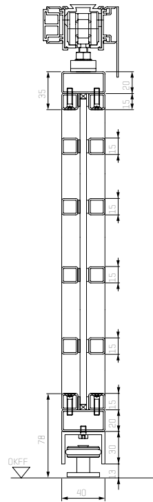
Vertikalschnitt 2-flügelige Stahl-Lofttür
