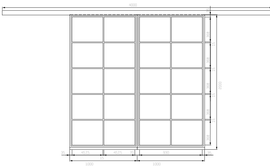
2-flügelige Stahl-Lofttür
