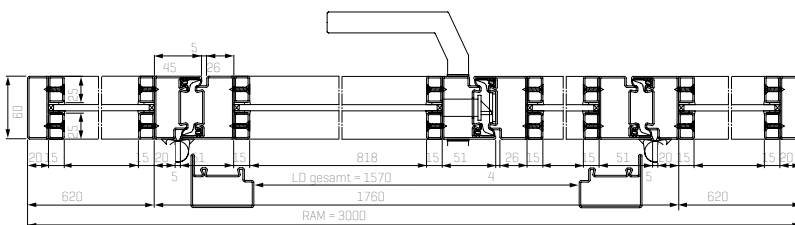
Horizontalschnitt 2-flügelige Stahl-Lofttür mit Seitenteilen
