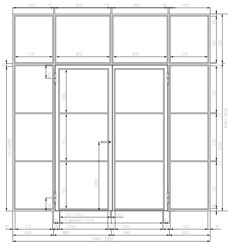
2-flügelige Stahl-Lofttür mit Seitenteilen und Oberlicht
