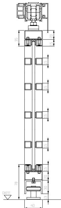
Vertikalschnitt 1-flüglige Stahl-Lofttür
