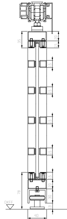
Vertikalschnitt 2-flügelige Stahl-Lofttür
