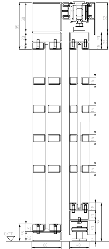
Vertikalschnitt 2-flügelige Stahl-Lofttür
