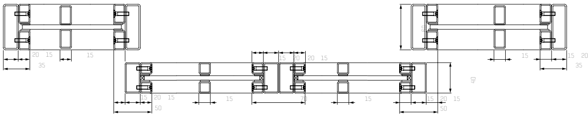
Horizontalschnitt 2-flügelige Stahl-Lofttür mit Seitenteilen
